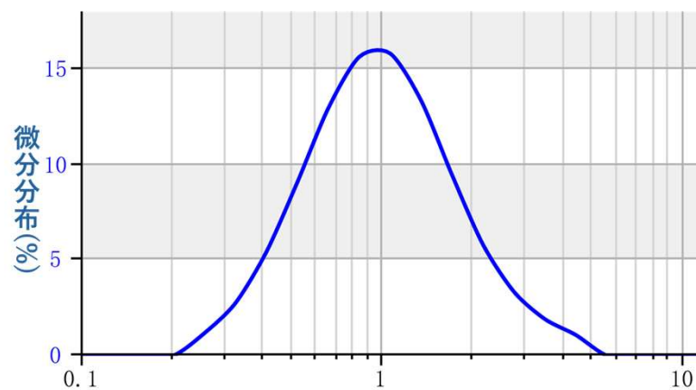
粒度分布図
